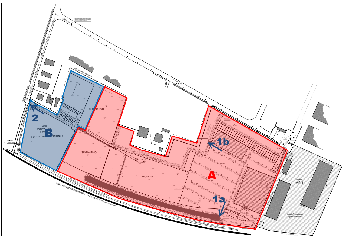
Figura 3 – Posizione dei tratti terminali dei collettori per il drenaggio delle acque meteoriche.
