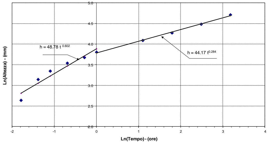
Figura 2 – Rappresentazione della curva di possibilità pluviometrica per il progetto dei collettori fognari.
