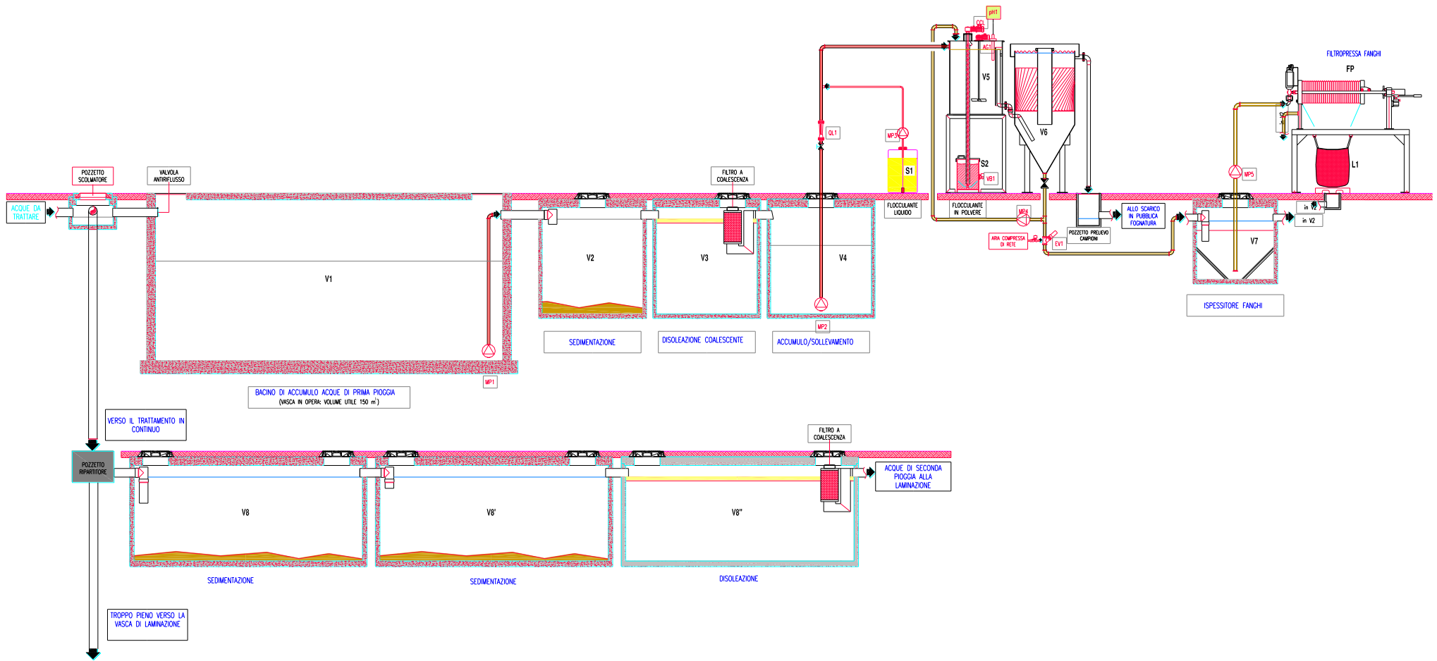
Figura 10 – Schema del sistema di trattamento delle acque meteoriche.
